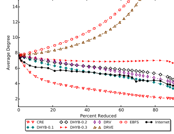
(b) CAIDA 2014-1998
